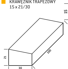
KRAWĘŻNIK TRAPEZOWY 15 x 21/30
